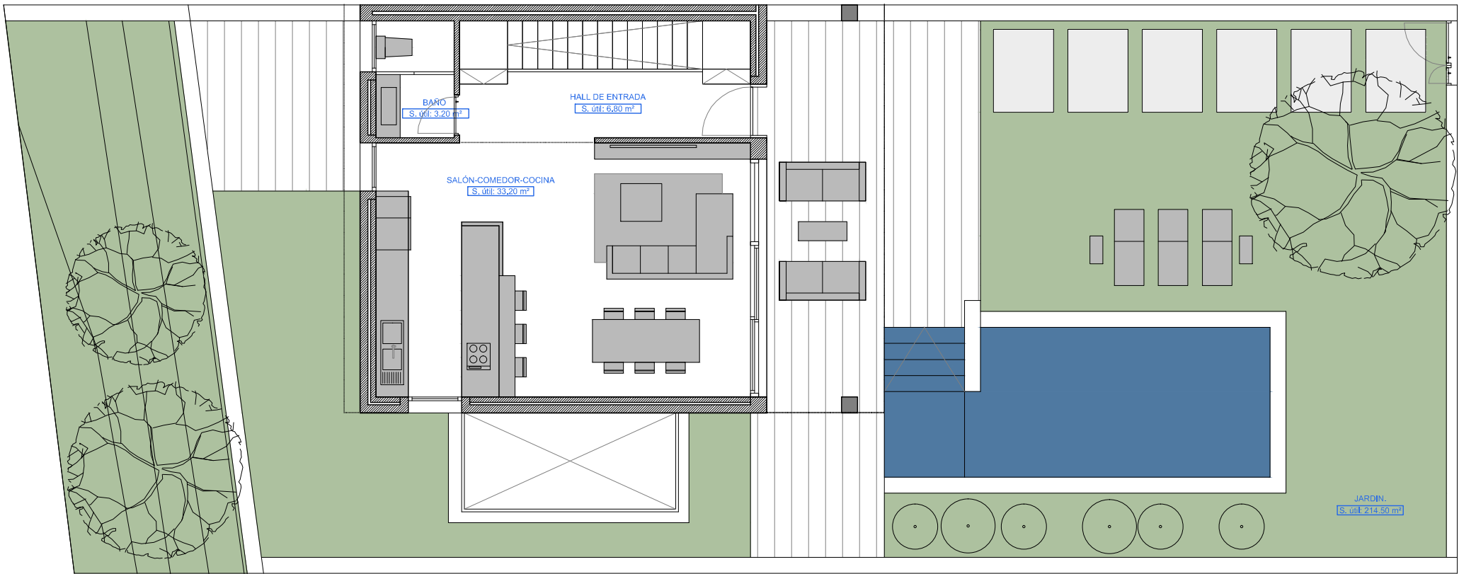
VIVIENDA TIPO C. Nivel +5.
