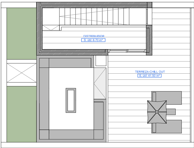
VIVIENDA TIPO C. Nivel +7.
