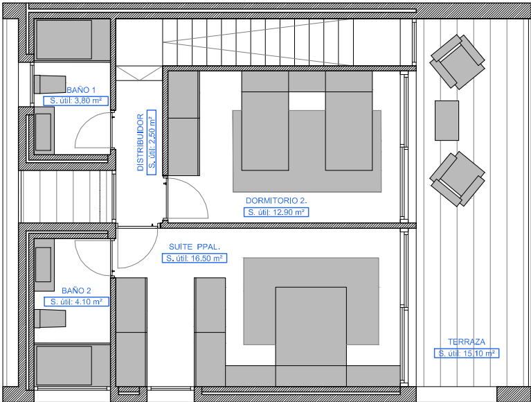
VIVIENDA TIPO C. Nivel +6.
