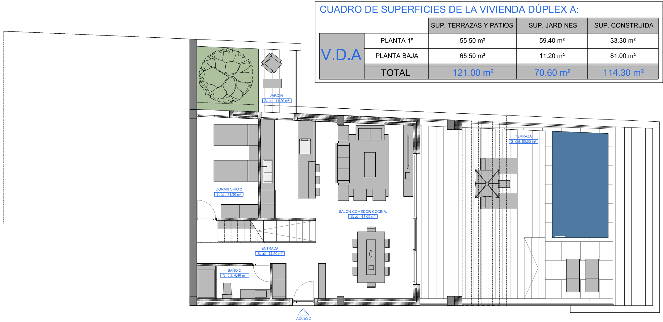
VIVIENDA DÚPLEX TIPO A. Nivel +4.
